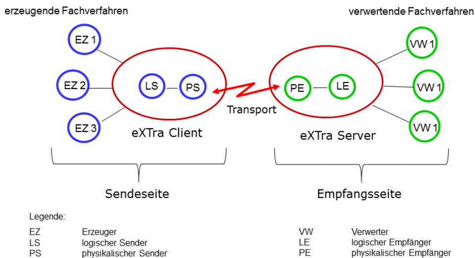
Bild 2: Das schematische Zusammenspiel der kooperierenden Fachverfahren mit eXTra für erzeugende Fachverfahren auf Senderseite und verwertende Fachverfahren auf Empfängerseite
